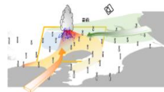
線状降水帯や局地豪雨の予測
