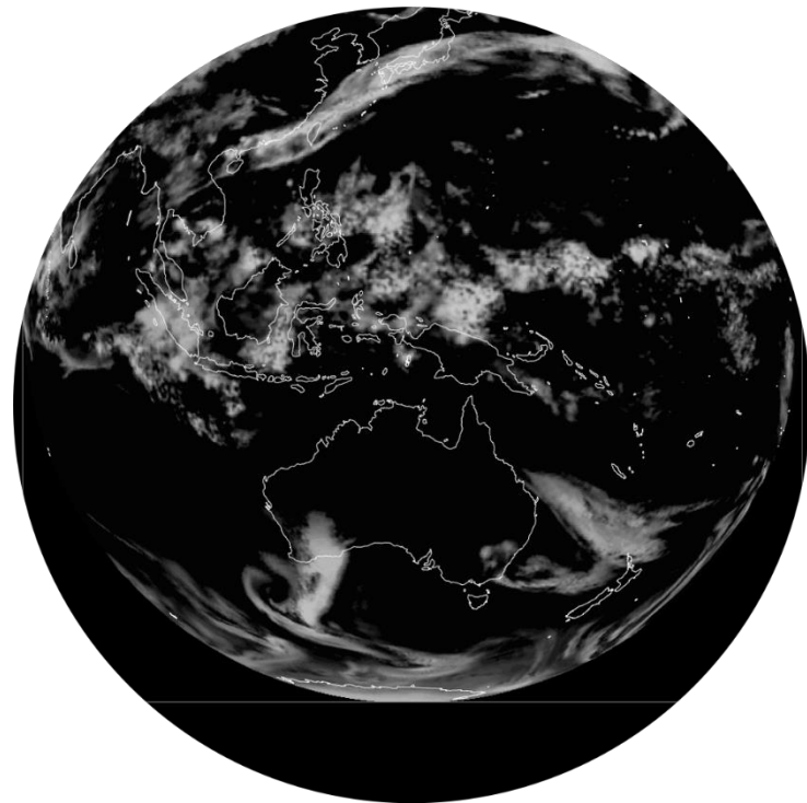
大気大循環モデル
